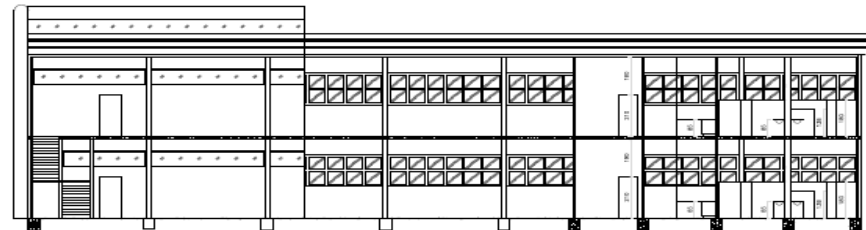
CORTES BB ESCALA 1:100
